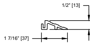
THRESHOLD ADD-ON DE3282-01_
